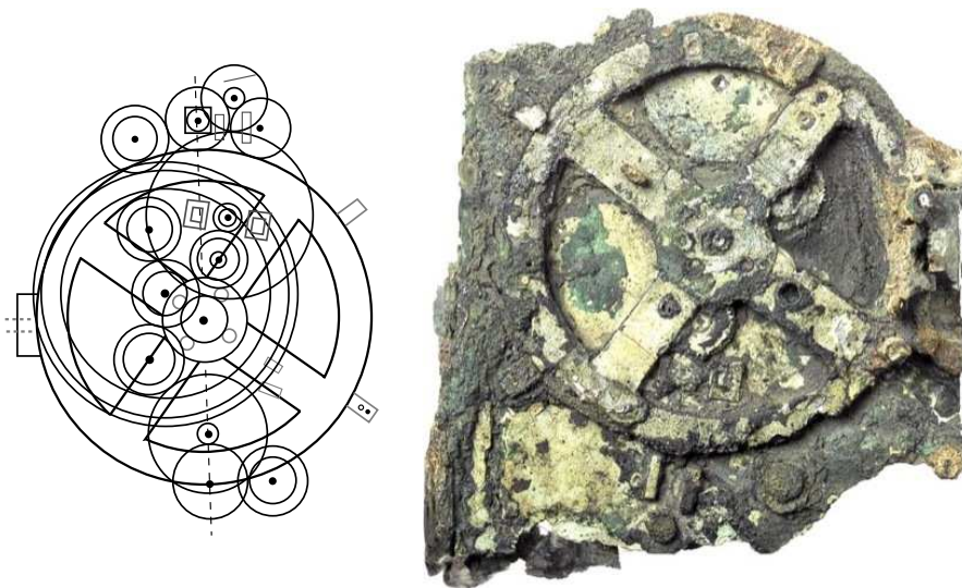
Figura 2. Mecanismo de Antikythera. Primer modelo de engranajes conocido, para determinar la posición de los planetas (la imagen es de Wikipedia).[3]
